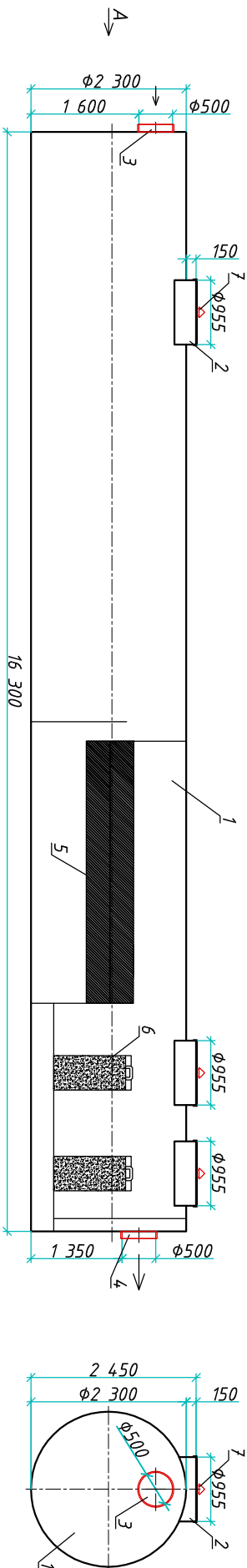
Разрез 1-1
